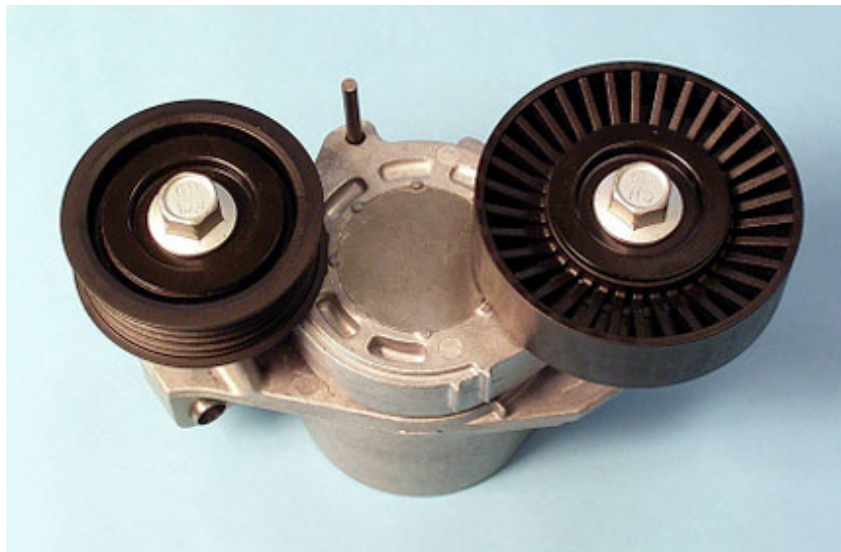
自動車用補機駆動システムに使用する オートテンショナー
