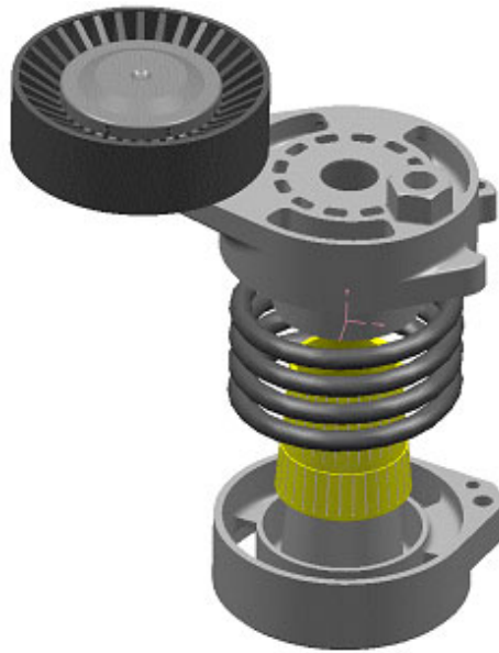
AUDI V6 2,4i に使用されている オートテンショナーの模式図
