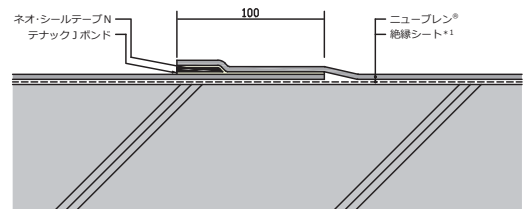
■接合部：NB-101HF/NB-101M
