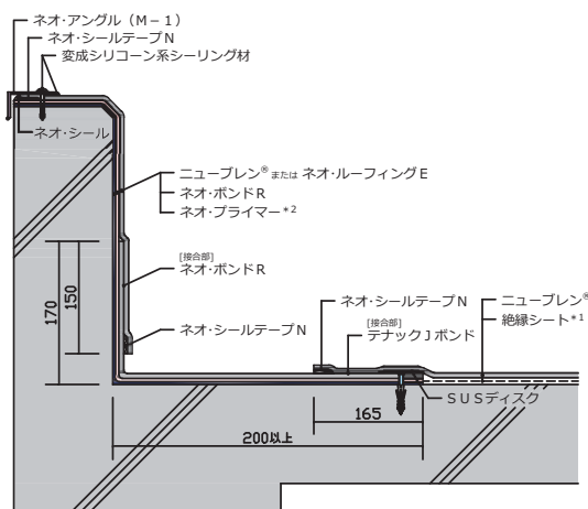
■NB-101MJ（周囲部は接着工法）
